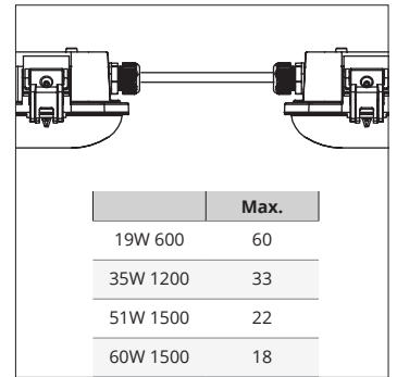
Doorvoerbedrading 5x2.5mm 2
